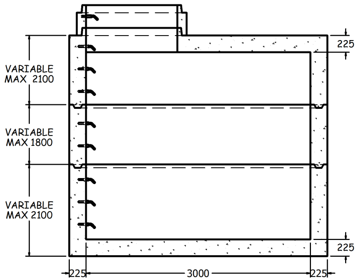
SECTION A-A 1:50
