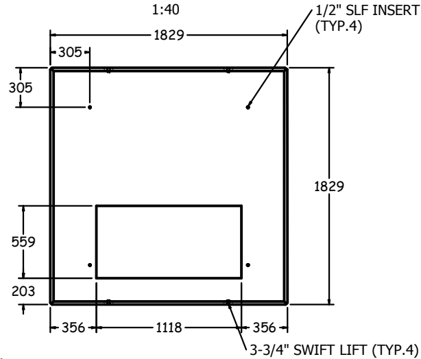
TOP VIEW LID 1:40
