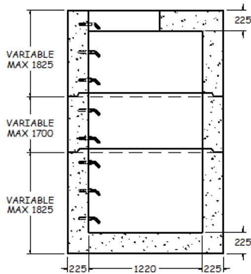
SECTION A-A 1:40
