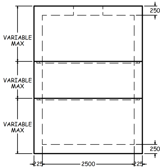
SECTION A-A 1:60
