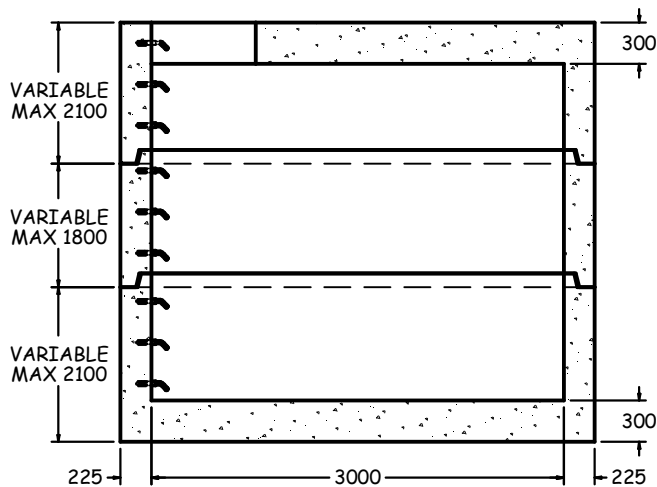
SECTION A-A 1:55
